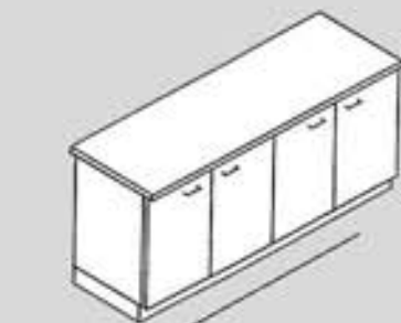
Modulo H - due doppia antina dim. L 180 x P 65 x H 87 cm
